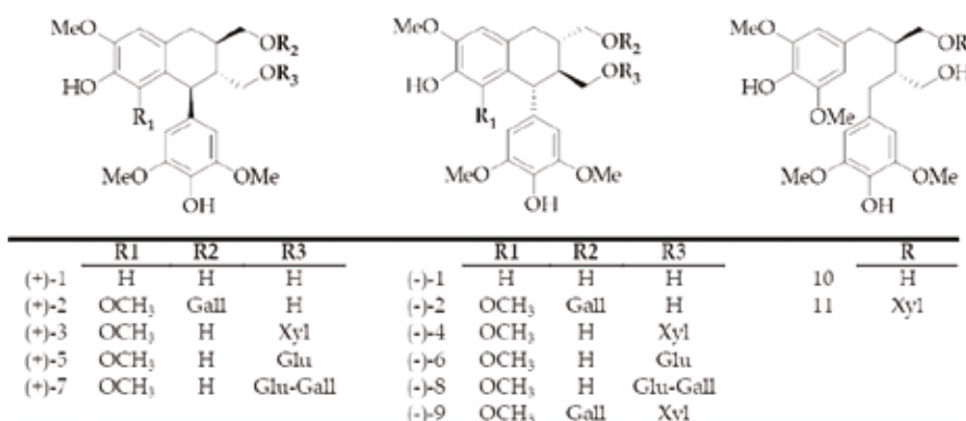
Figure 1 : Structure chimique des lignanes 1 à 11. Xyl, Glu et Gall correspondent, respectivement, au β-xylopyranose, β-gluco-pyranose et galloyle.
