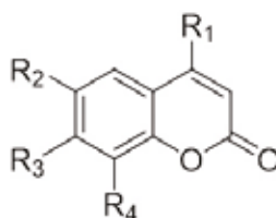
Figure 3 : Structure chimique des six coumarines ciblées.
