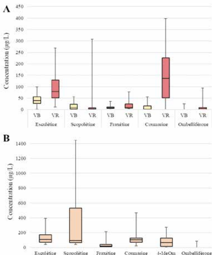
Figure 4 : Variations des concentrations de l'esculétine, la fraxétine, la scopolétine, l'ombelliférone, la coumarine et de la 4-méthylombelliférone (4-Meom) dans 90 vins commerciaux (A) 28 eaux-de-vie commerciales (B)
